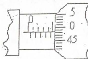
螺旋测微器
